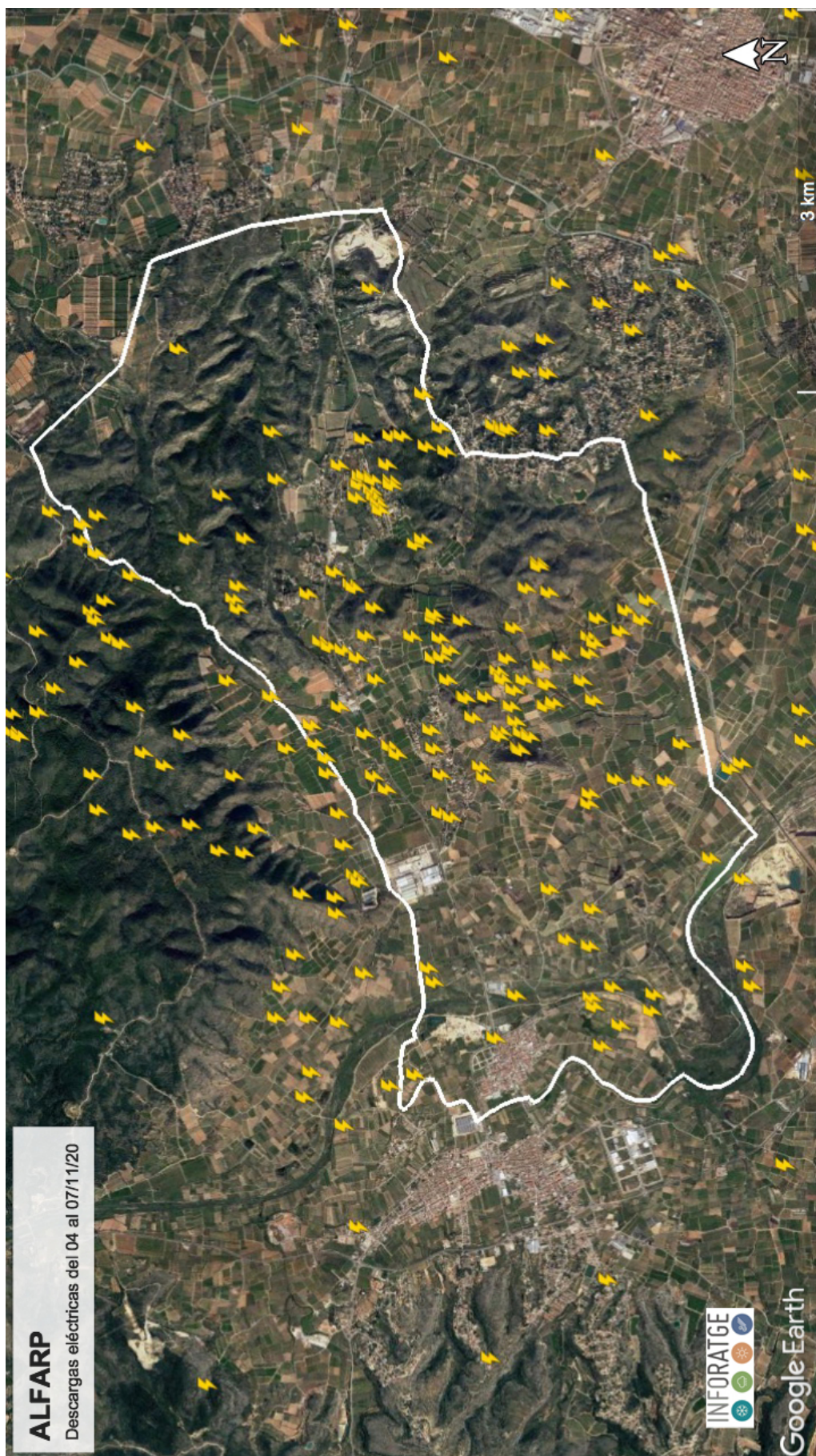
Geolocalización de las descargas eléctricas ~ nube-tierra registradas en el término municipal de ALFARP y alrededores entre los días 04 y 07/11/20 Fuente descargas eléctricas: AEMET Agencia Estatal de Meteorología // Cartografía: Instituto Geográfico Nacional de España
